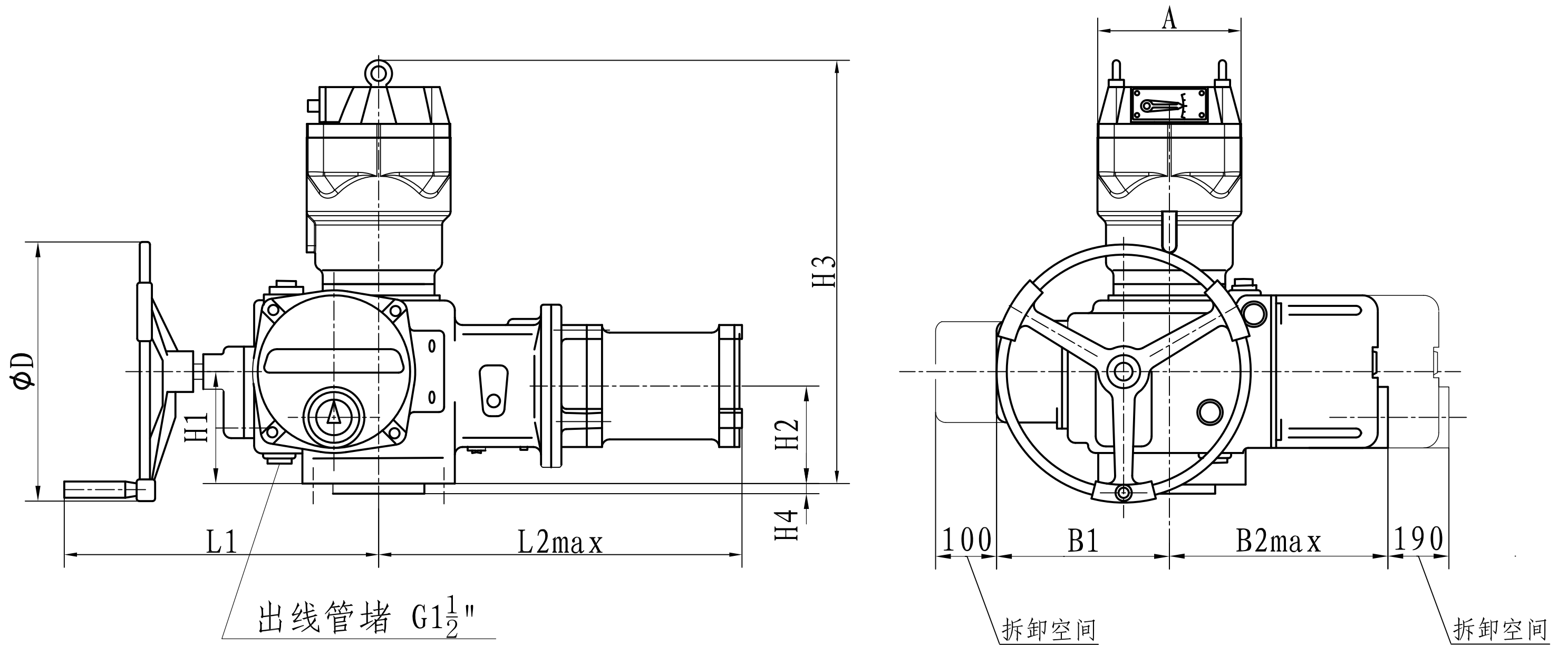
SCD00-2外形尺寸
